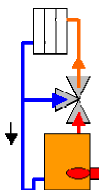
Ενδεικτική λειτουργία τρίοδης βάνης ευθείας ροής
